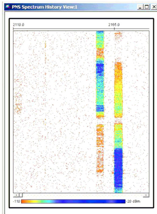
Fig6.- Característica temporal de la densidad de potencia espectral en la banda Downlink en UMTS. Se pueden ver 3 canales UMTS activos y una interferencia CW transitoria.
