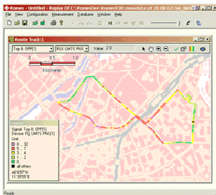
Fig1.- El mapa de análisis de Pilot pollution muestra el número de señales piloto ( HPP \cong Hard Pilot Pollution ó SPP \cong Soft Pilot Pollution, parámetros calculados a partir de la relación (RSCP_{bestserver}/RSCP_n) ), de las estaciones base dentro de un canal, que exceden un valor umbral de potencia configurable.
