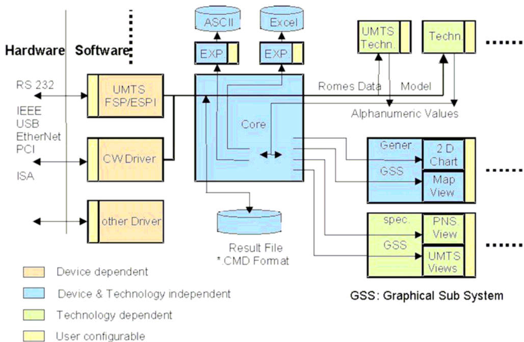
Fig9.- Concepto software medida R&S ROMES
