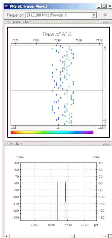
Fig2.- Fading “Birth death” 3GPP , especificado en los conformance tests de móviles, generado por el generador de señales R&S SMU200A y medido con el PN Scanner R&S TSMU. Modo de representación Tracer SC View (Respuesta impulsiva y diagrama waterfall para hacer un seguimiento de un código de scrambling )
