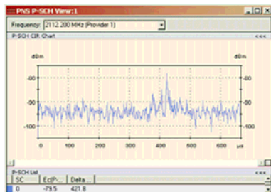
Fig4a.- Secuencia de sincronización primaria filtrada de una señal UMTS por medio de un correlador estándar
